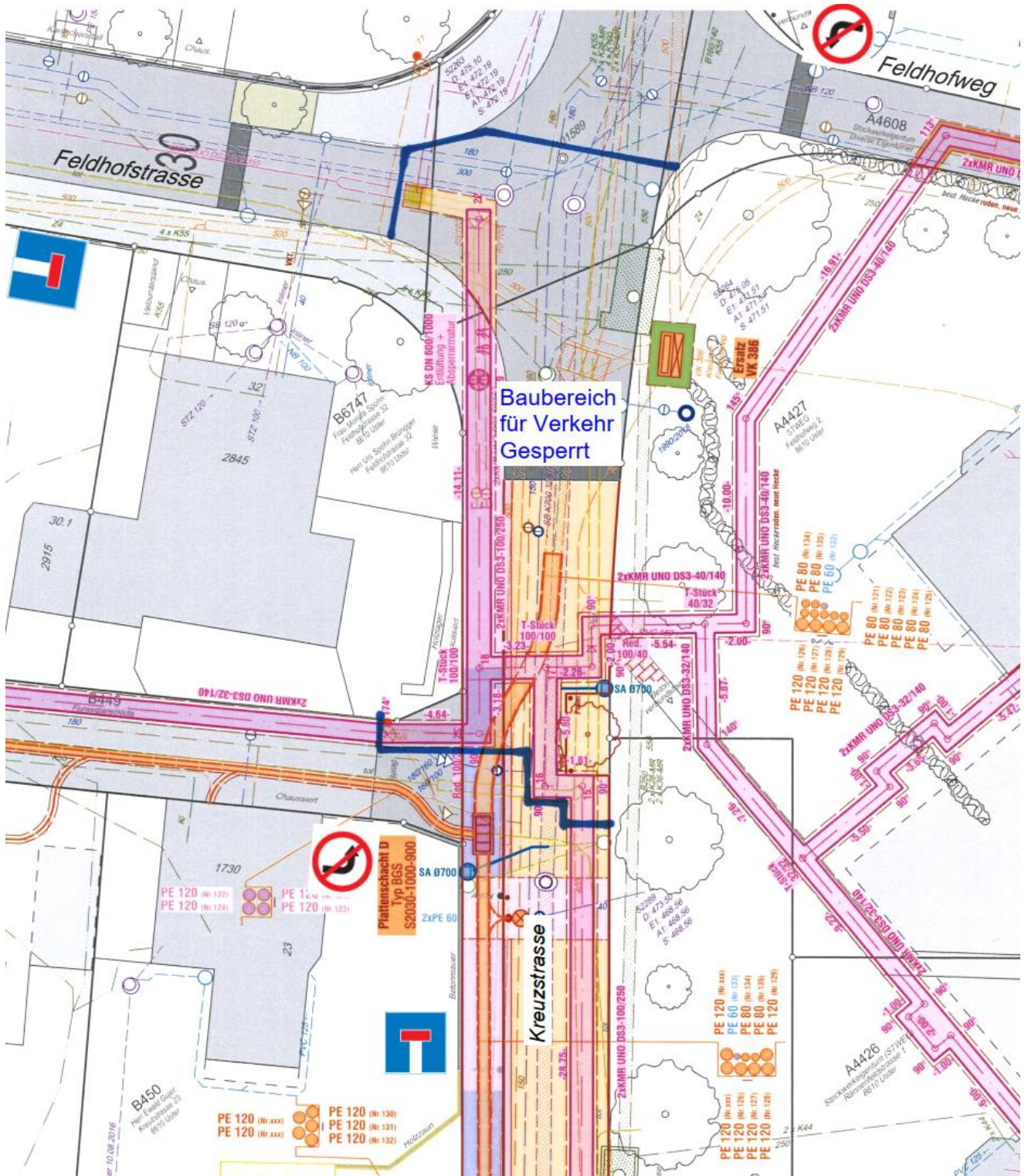
Übersichtsplan Baubereich
