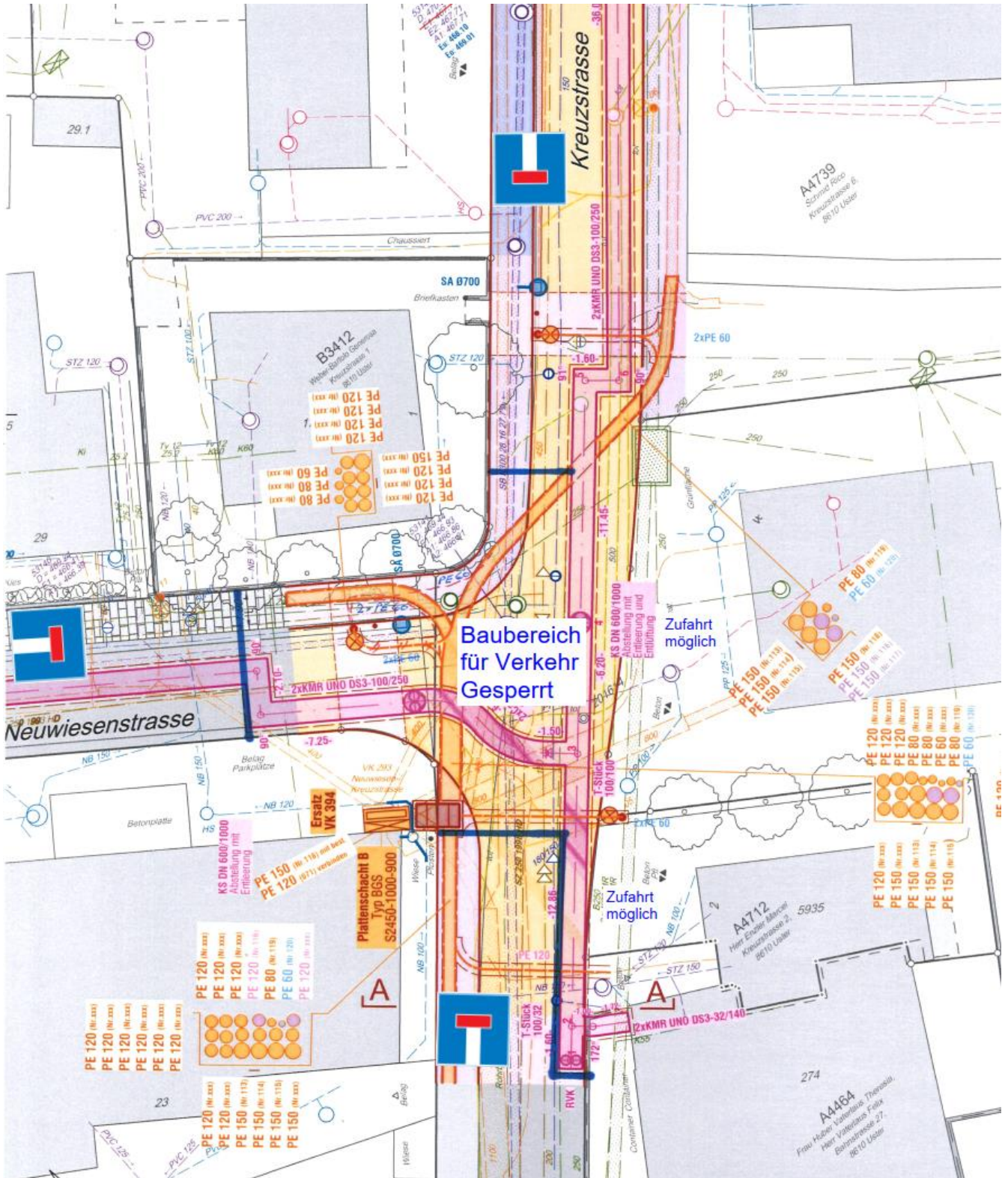
Übersichtsplan Baubereich
