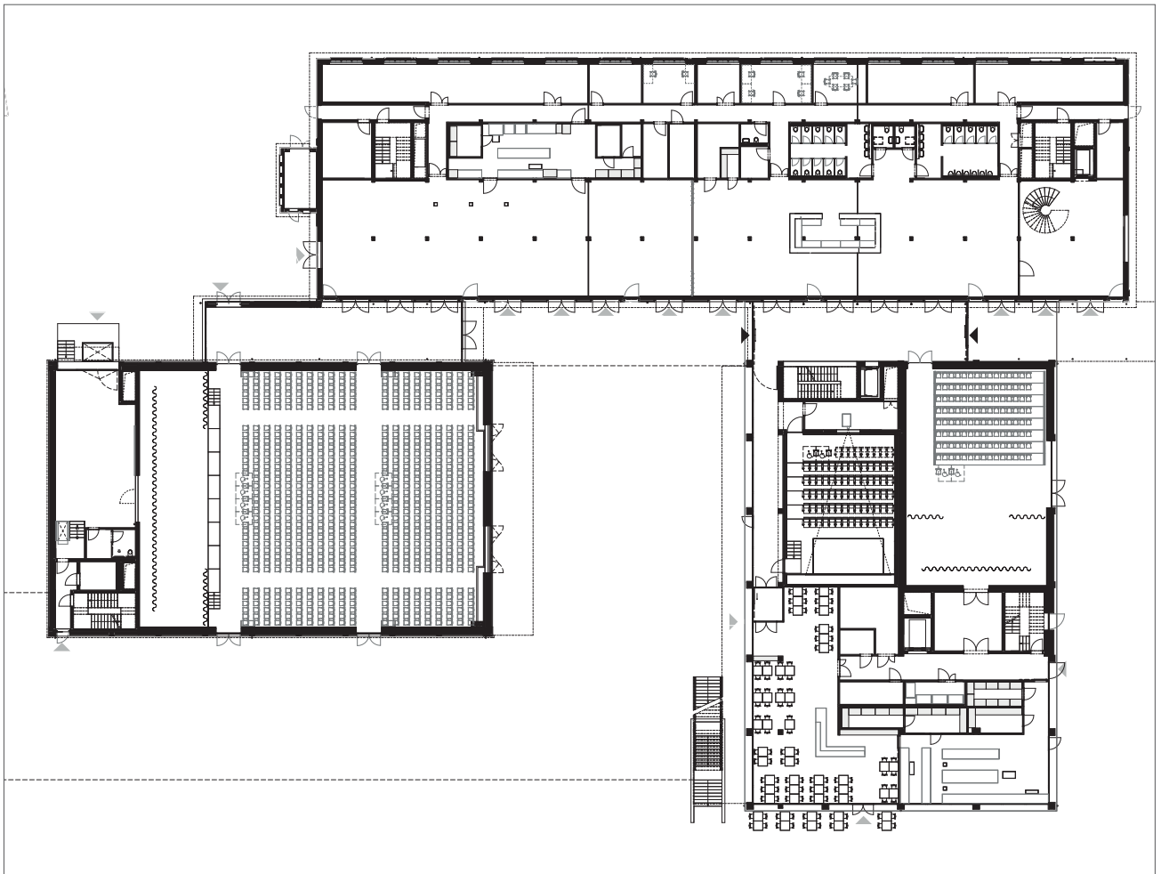
Abbildung 4: Grundrissplan; links: Grosse Saal, Mitte: Zeughaus K2 mit Foyer, rechts: Regal mit Kino, kleiner Bühne und Gastronomie
